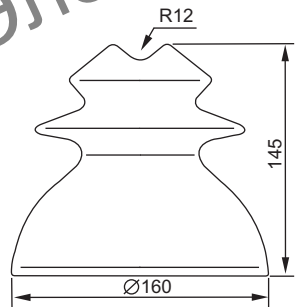
ЗАМЕНЯЕМЫЙ ШТЫРЕВОЙ ФАРФОРОВЫЙ ИЗОЛЯТОР ШФ-10
