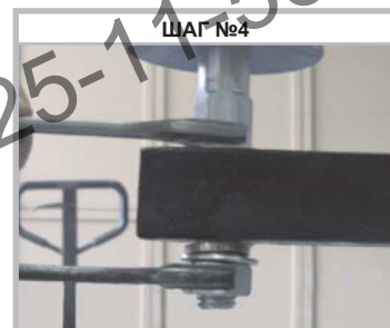
ШАГ №4 Закрепите изолятор на траверсе, при помощи двух ключей
