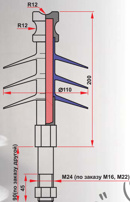
ЗАМЕНЯЕМЫЙ ШТЫРЕВОЙ ФАРФОРОВЫЙ ИЗОЛЯТОР ШФ-10
