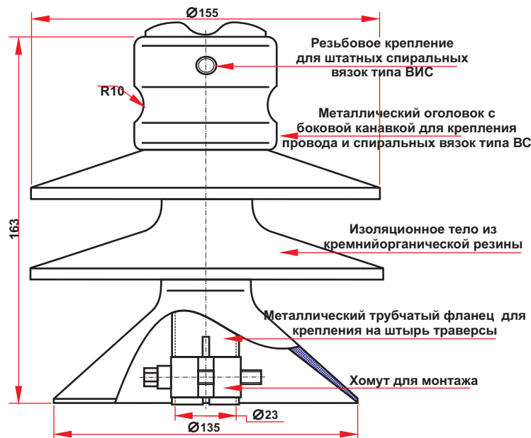
ИЗОЛЯТОР ПОЛИМЕРНЫЙ ШТЫРЕВОЙ ШПУ-20 УХЛ1
